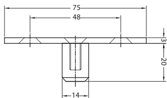
Pivot haut pour plinthe haute FRP02 Top pivot for top door rail FRP02
